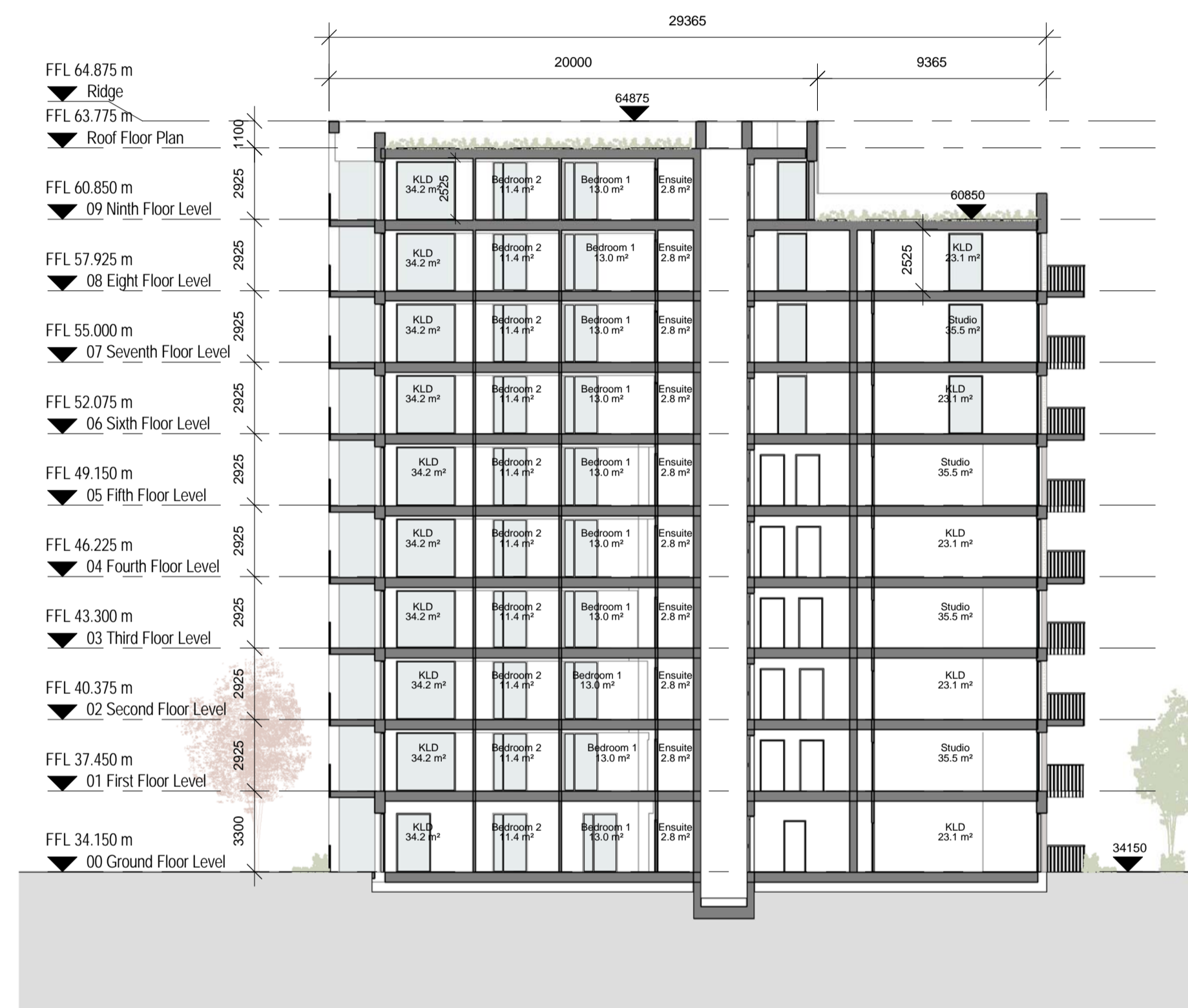
1 Cross Section B 1 : 200
